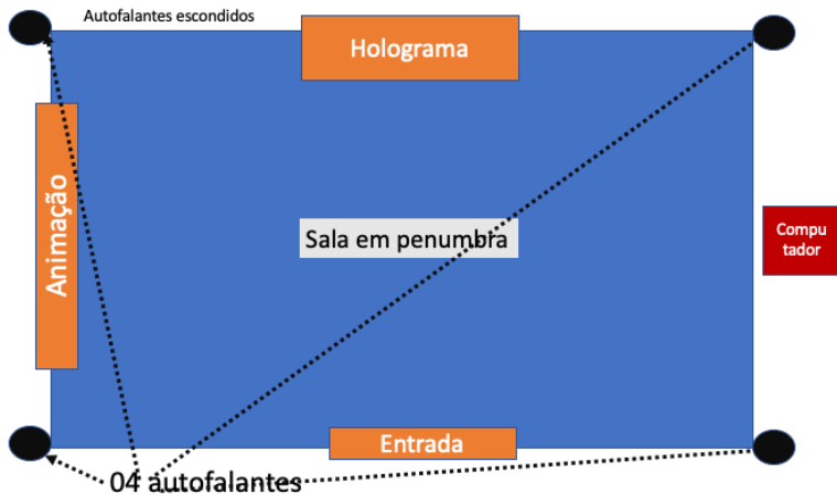
Planta baixa da instalação "Modalities Est Agnus Dei."
